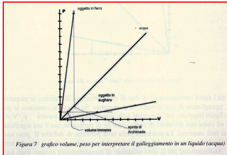
Figura 7 grafico volume, peso per interpretare il galleggiamento in un liquido (acqua)
